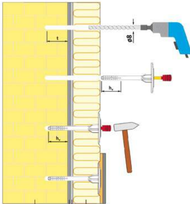
забивной дюбель
