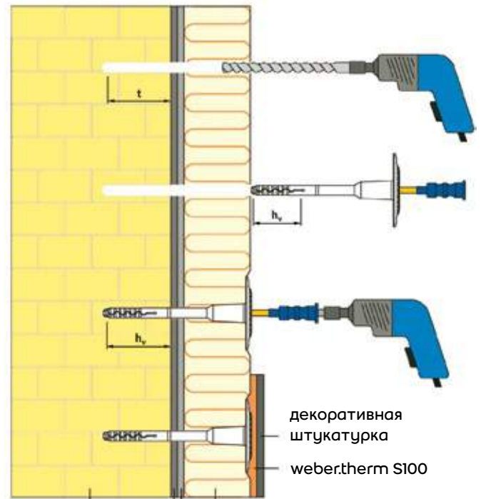
винтовой дюбель
