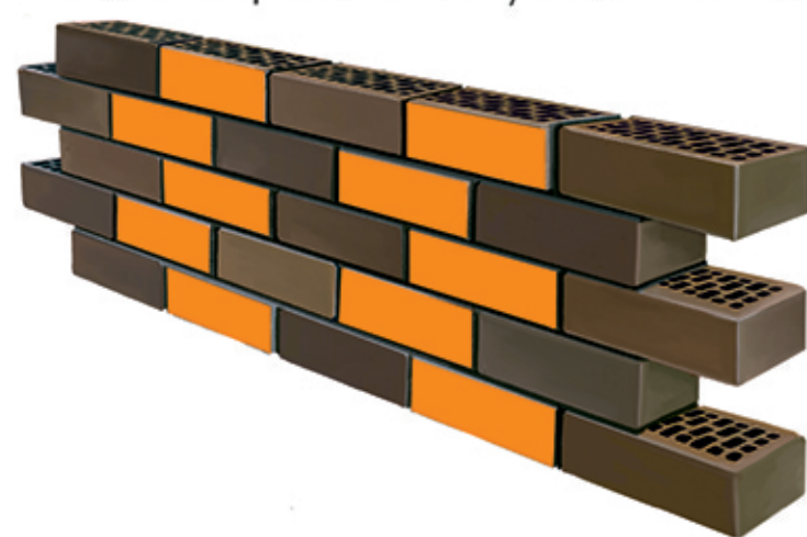
4 ЛОЖКОВАЯ КЛАДКА СМЕЩЕНИЕ НА 1/4 КИРПИЧА
