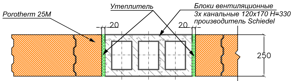
Перевязка стены из Porotherm 38 с вентиляционным 2х канальным блоком Schiedel
