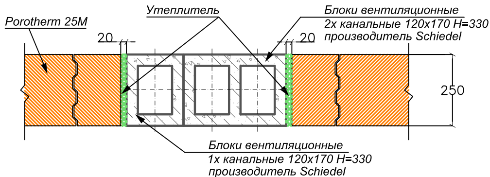
Перевязка стены из Porotherm 25M с вентиляционным 3х канальным блоком Schiedel
