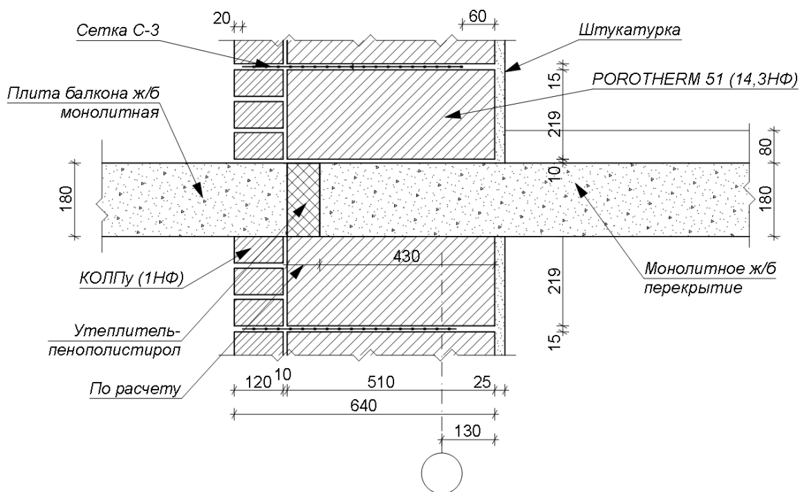
В - В
