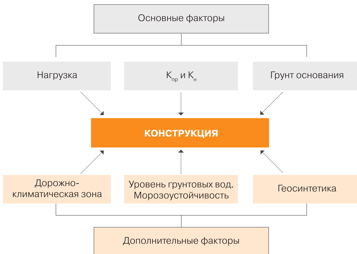
Рисунок 11. Факторы, определяющие вид конструкции
